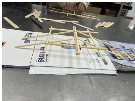
使用竹筷子搭建達文西橋
